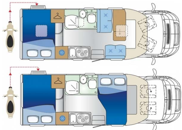
Heckgarage
